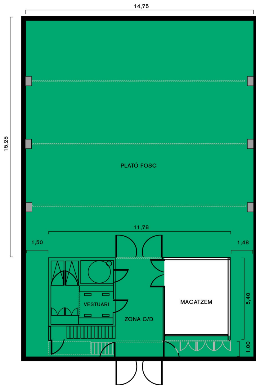
SALA RICSON - PLANTA BAIXA
