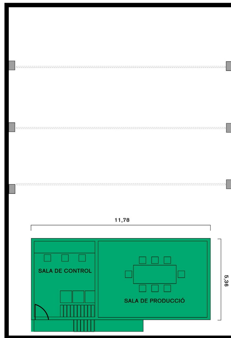
SALA RICSON - PLANTA ALTA
