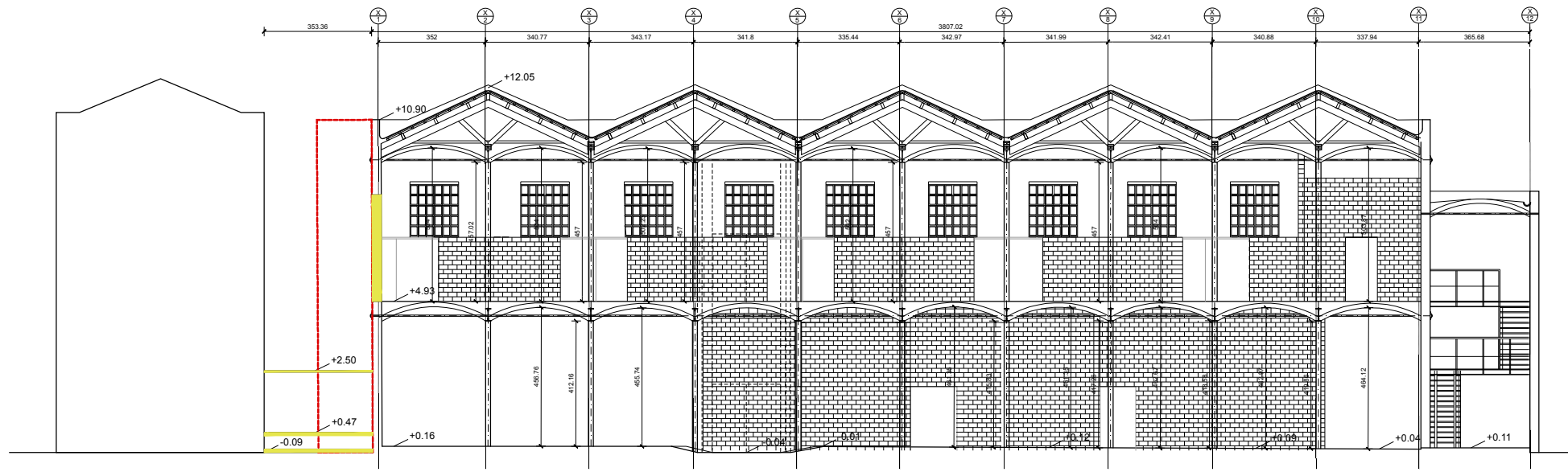
SECCIÓ LONGITUDINAL ST 1
