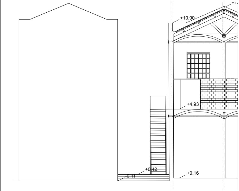
SECCIÓ LONGITUDINAL ST 1
