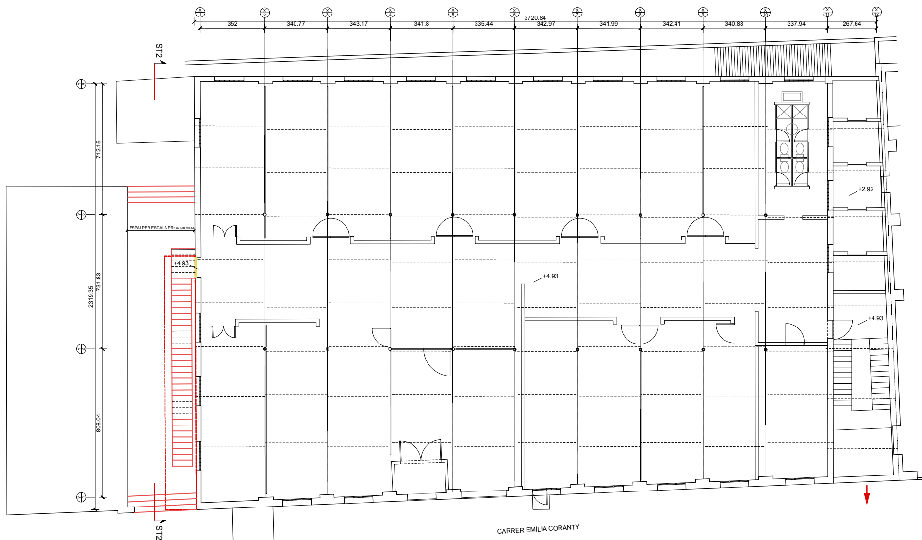
PLANTA PRIMERA
