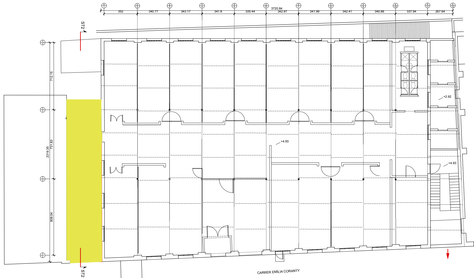
PLANTA PRIMERA
