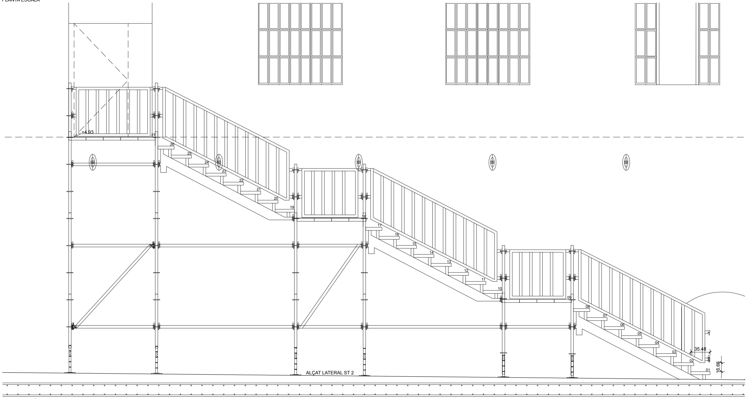
ALÇAT-SECCIÓ ESCALA
