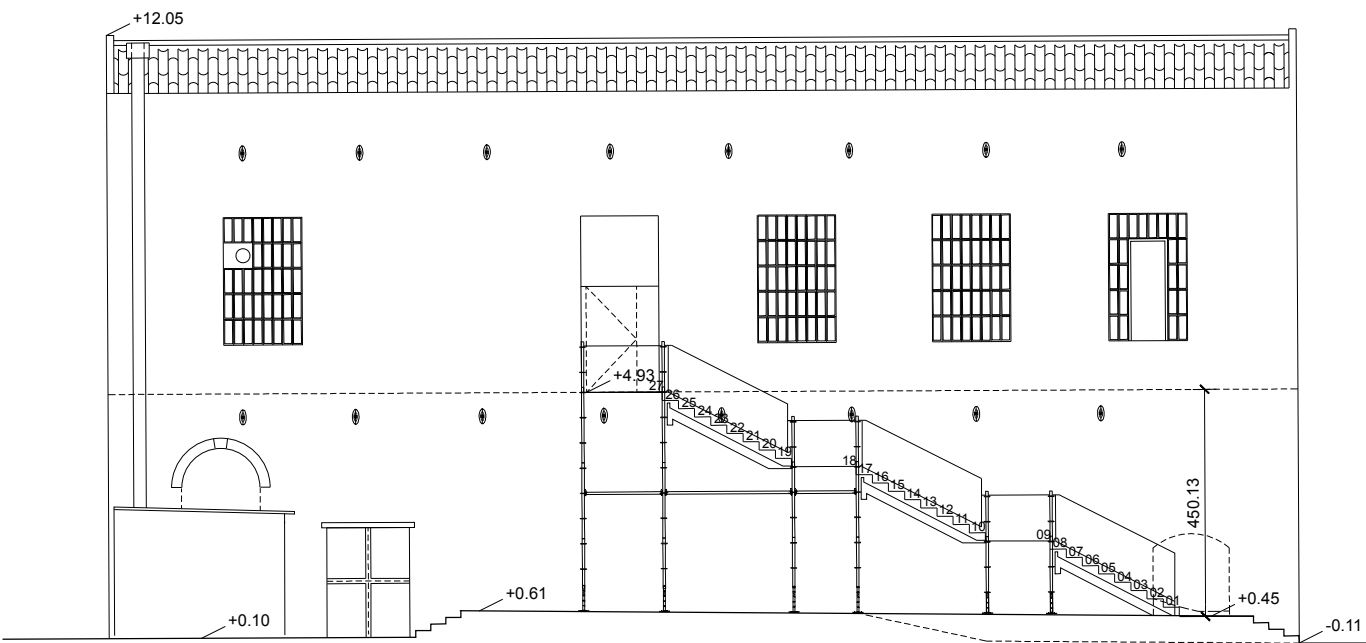
ALÇAT LATERAL ST 2
